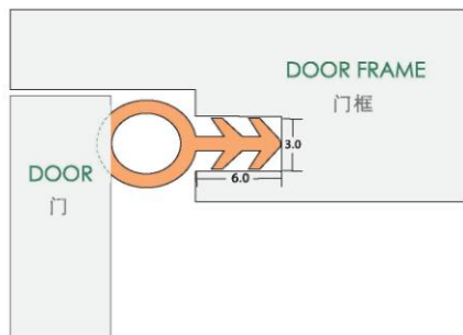
安装效果图 Installation diagram
