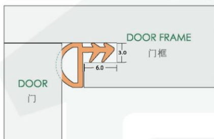
安装效果图 Installation diagram
