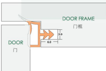
安装效果图 Installation diagram
